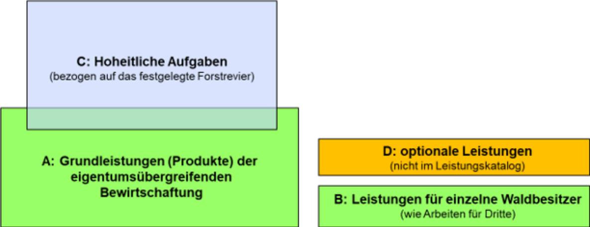
Abbildung 1: Leistungsmodell
